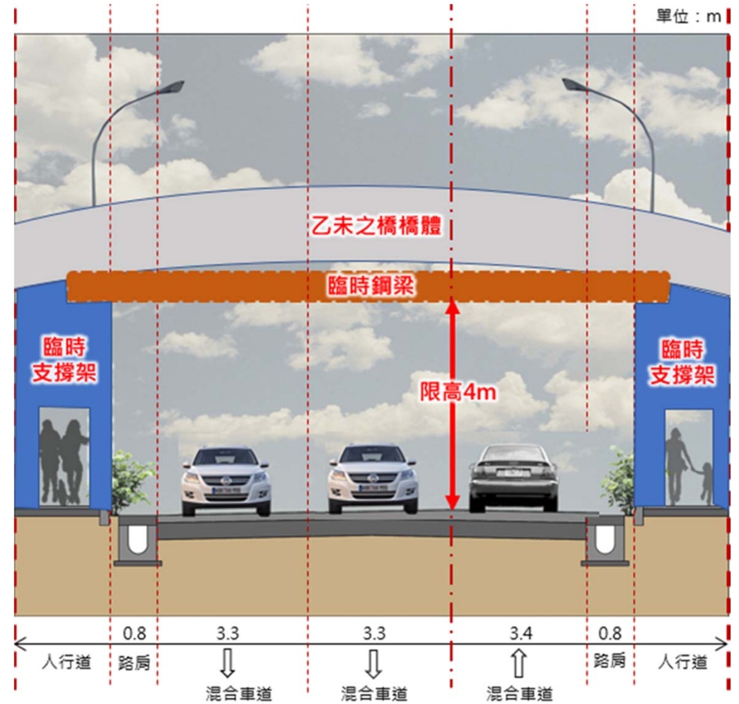
限高示意圖
