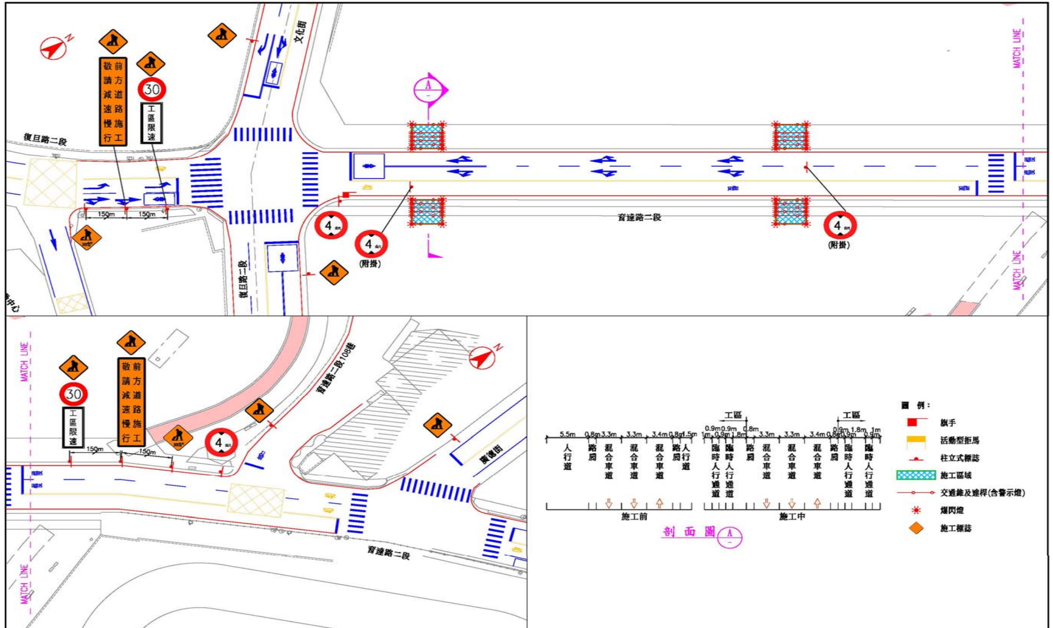
交通維持佈設圖
